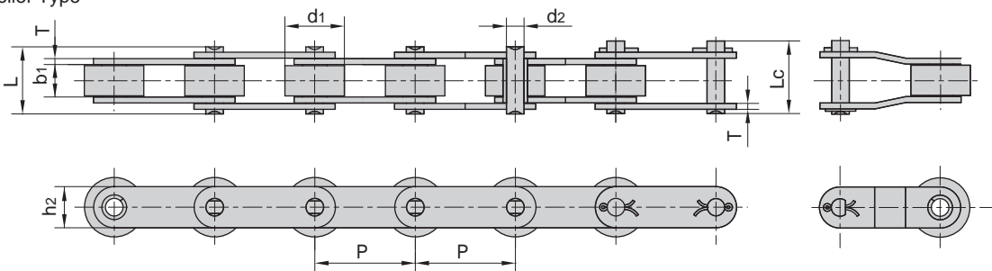
大滚子型 Large Roller Type
